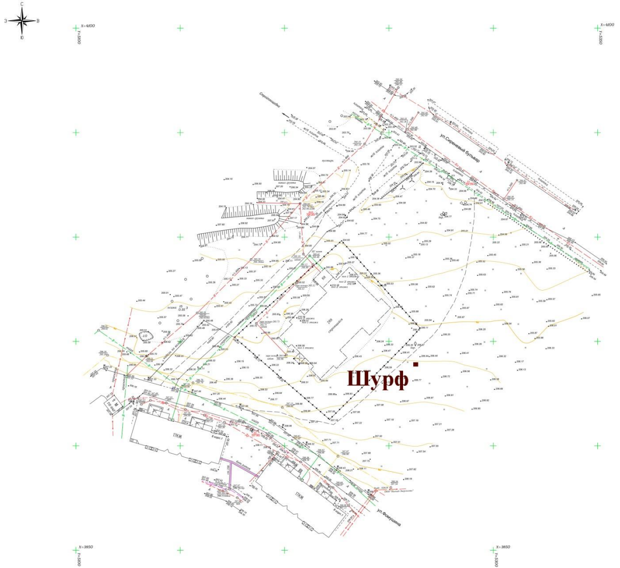
Рис. 16. Земельные участки с кадастровыми номерами 40:26:000374:1722, 40:26:000374:2332 для строительства объекта «Дошкольная образовательная организация на 325 мест», по адресу: г. Калуга, ул. Сиреневый бульвар». С обозначением места шурфа.
